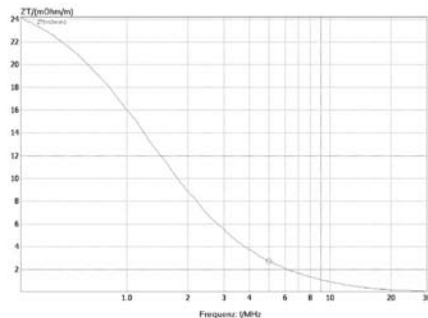
Kopplungswiderstand|Coupling resistance
